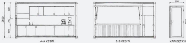
A-A KESİTİ
