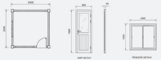
KAPI DETAYI
